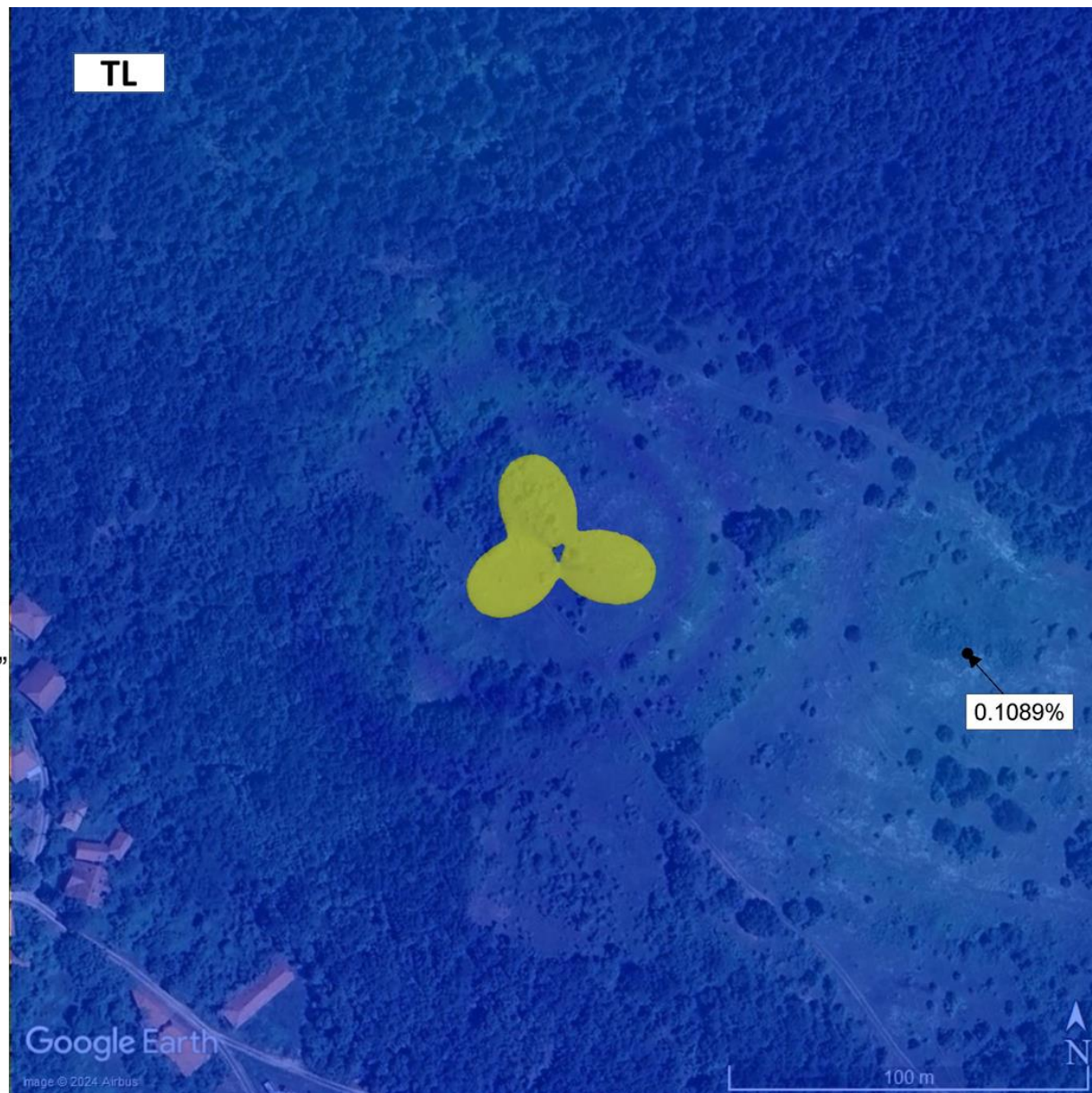
Слика 4.6. Фактор изложености на тлу када сви радио-системи оператора Telekom Srbija раде максималним капацитетом
