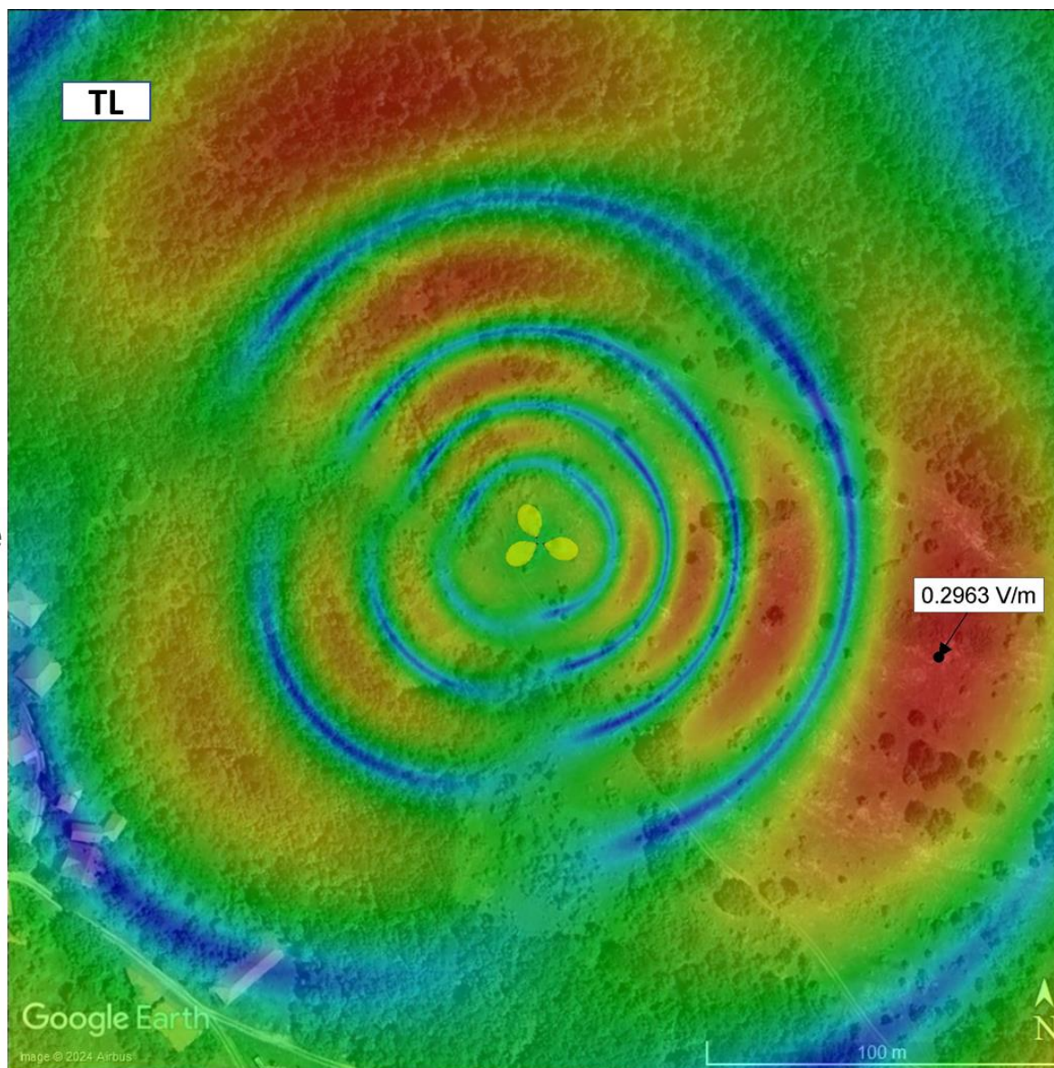
Слика 4.2. Јачина електричног поља на тлу када радио-систем GSM900 оператора Telekom Srbija ради максималним капацитетом
