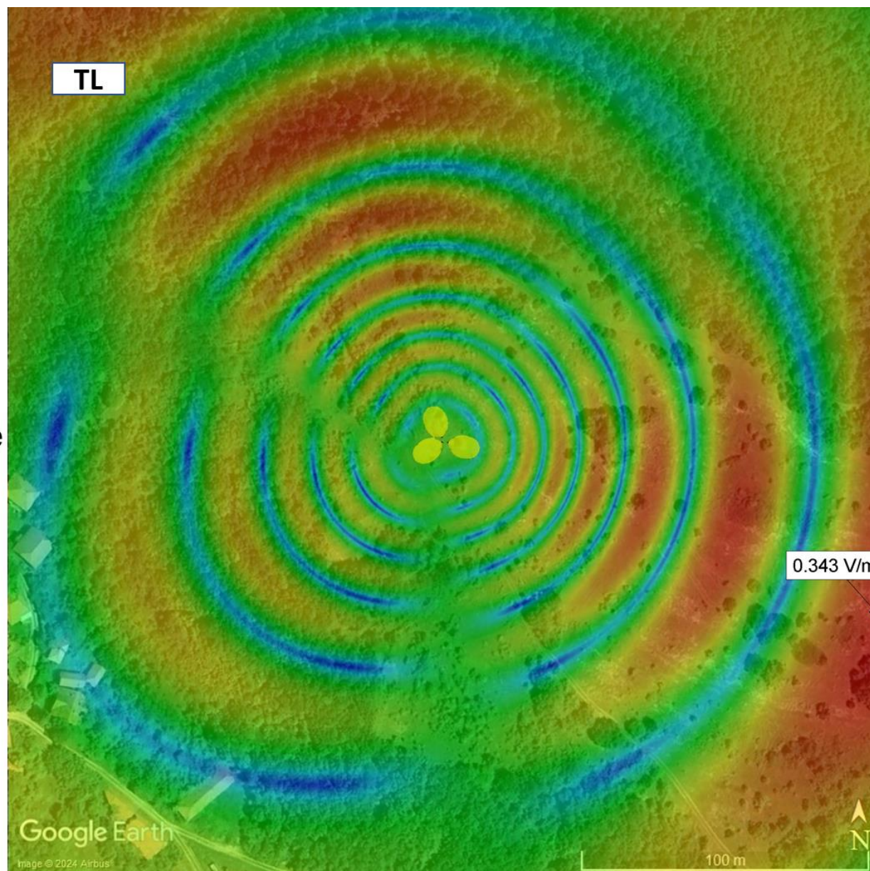
Слика 4.5. Јачина електричног поља на тлу када радио-систем LTE2100 оператора Telekom Srbija ради максималним капацитетом
