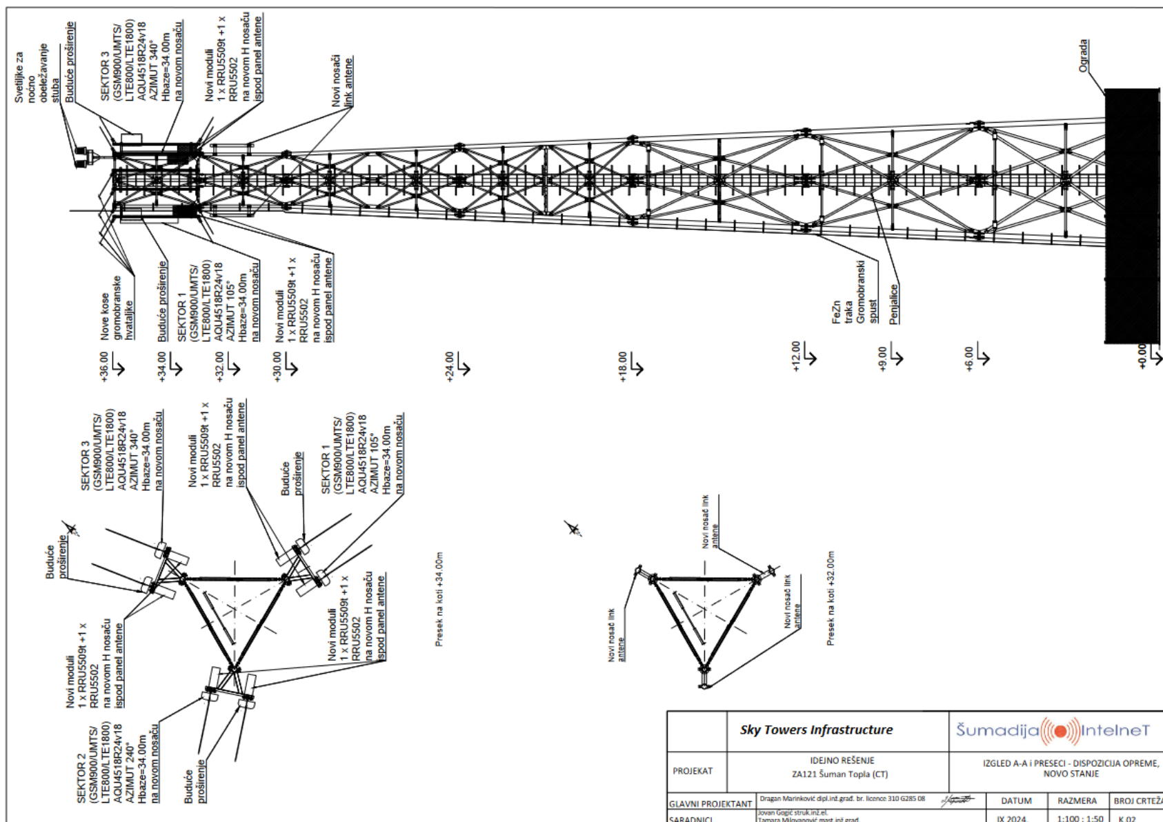
Слика 8.2. Идејно решење – изглед А-А и пресеци - диспозиција опреме
