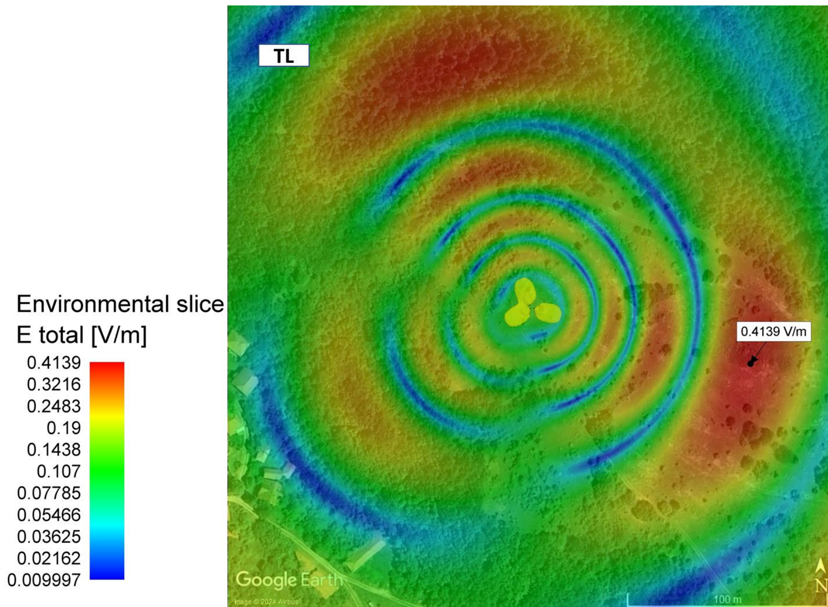
Слика 4.3. Јачина електричног поља на тлу када радио-систем LTE800 оператора Telekom Srbija ради максималним капацитетом
