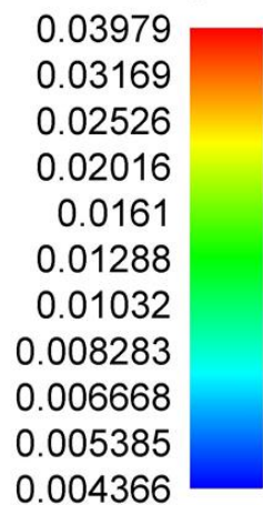
Слика 4.7. Јачина електричног поља унутар објекта када радио-систем GSM900 оператора Telekom Srbija ради максималним капацитетом
