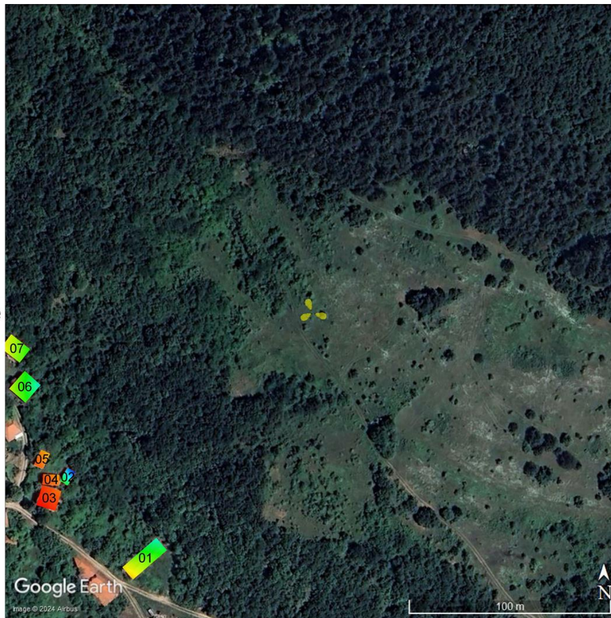
Слика 4.8. Јачина електричног поља унутар објекта када радио-систем LTE800 оператора Telekom Srbija ради максималним капацитетом
